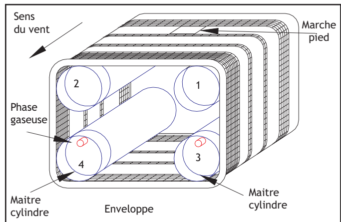
Positionnement correct des maîtres-cylindres ▲
