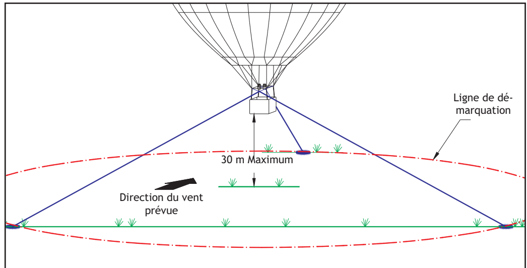
▲ Amarrage correct d'un ballon captif
