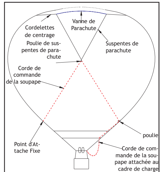
▲ Arrangement interne du parachute
