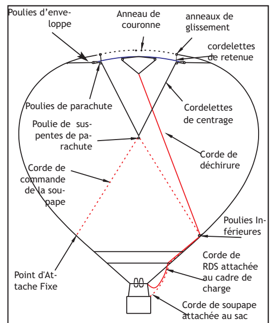
▲ Système de Dégonflement Rapide Arrangement Interne
