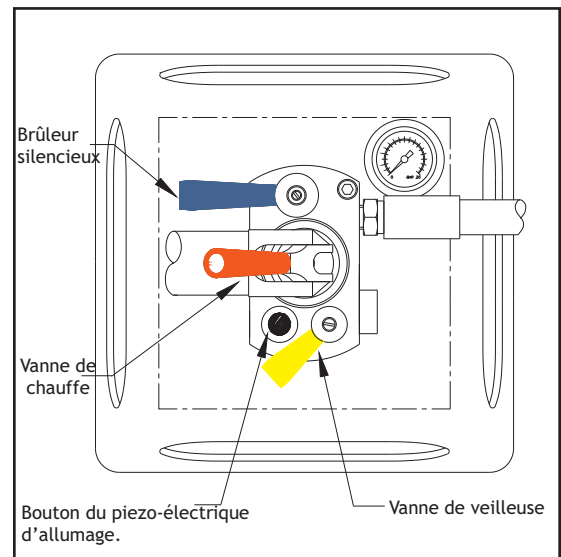
▲ Shadow / Stealth, Disposition des commandes
