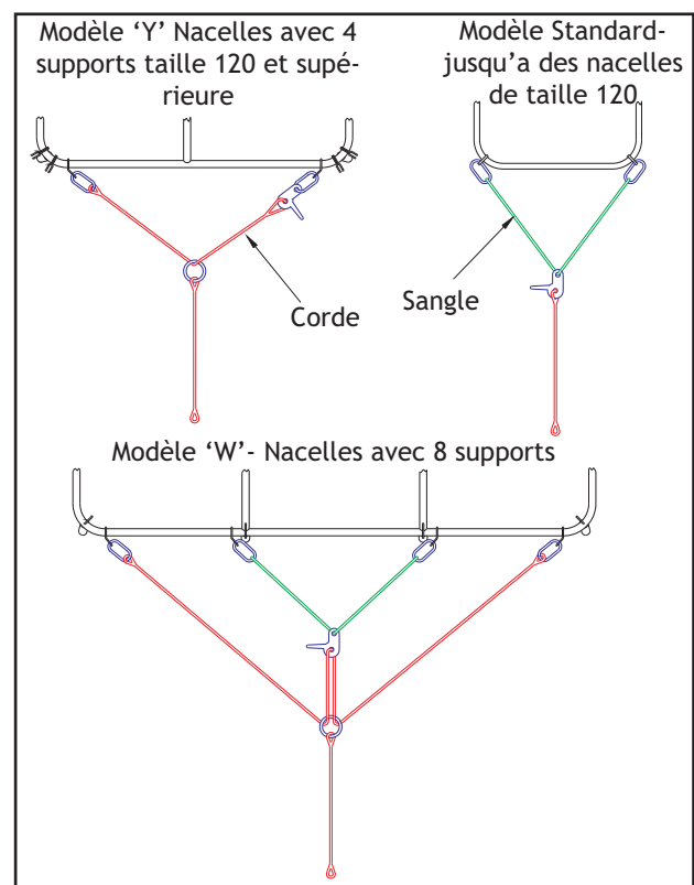
▲ Systèmes de largage
