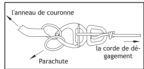
▲ Dispositif d'accrochage
