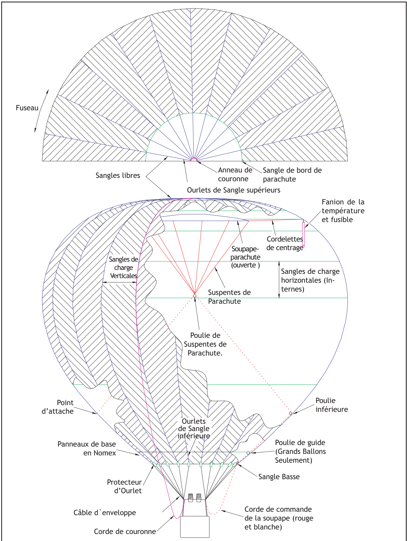
▲ Description typique d'enveloppe
