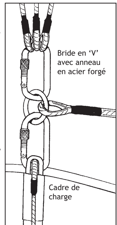
▲ Fixation de Bride en 'V'
